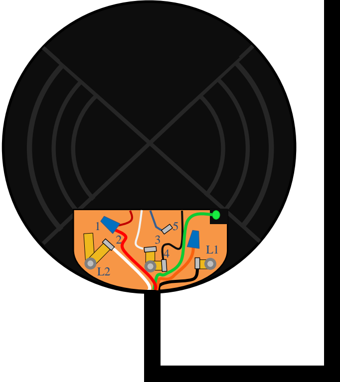
230 Volt Configuration
